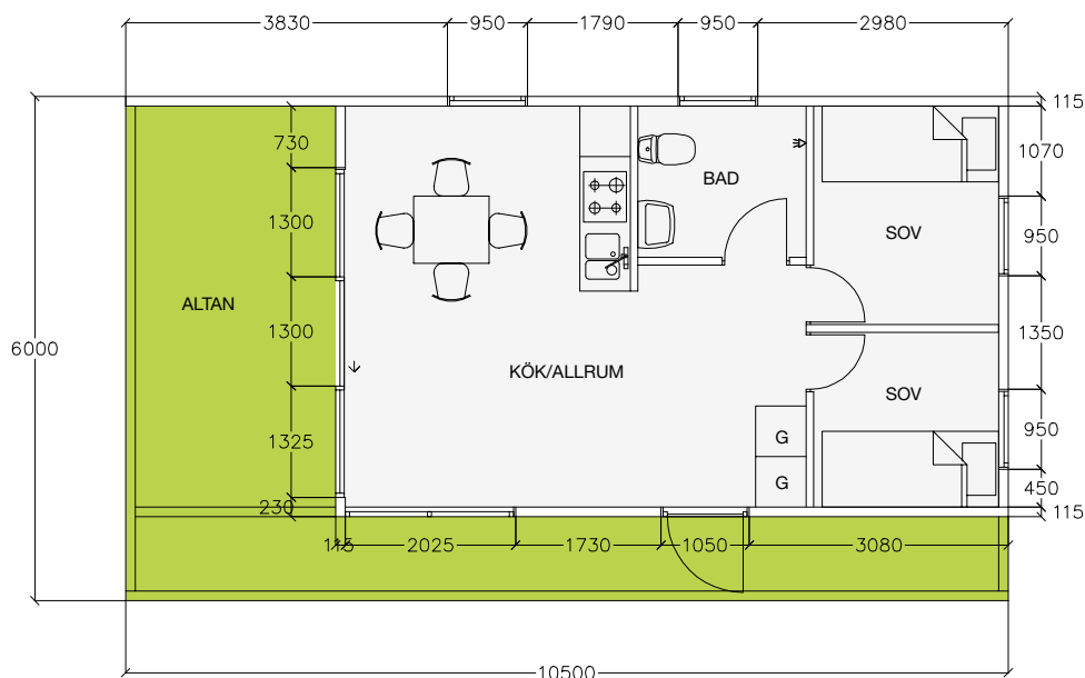
Plan 1:100
